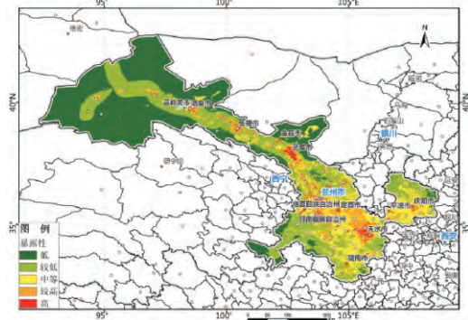
图2 甘肃省地质灾害暴露性空间分布图
