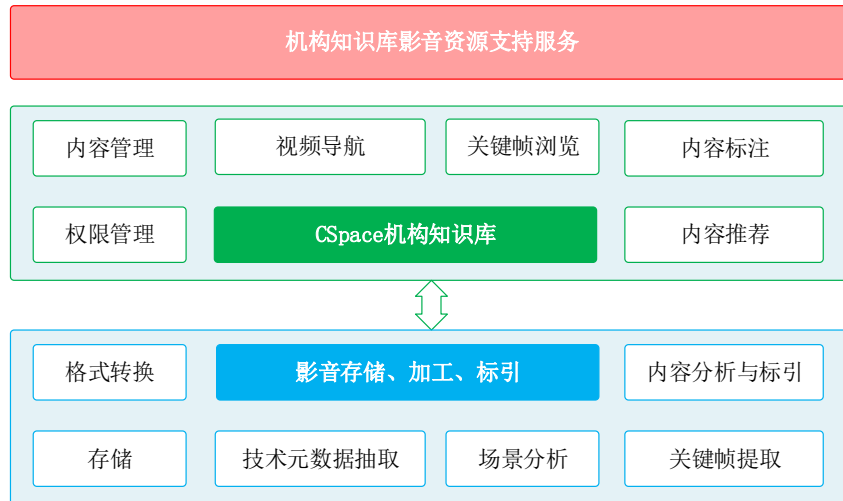
图 1 机构知识库影音资源支持功能框架
