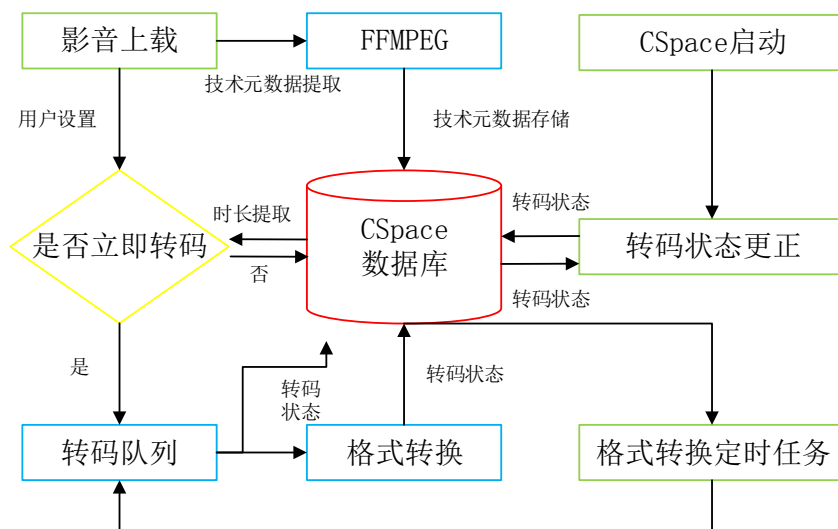
图 5 CSspace 影音格式转换机制
