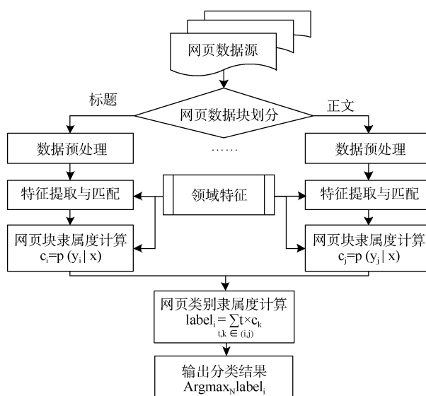
图 1 半监督网络科技信息分类模型框架
