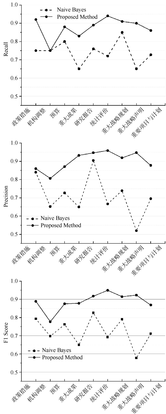
图 3 贝叶斯分类方法与本文方法的结果比较
