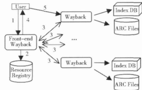
图 4 SDSC 全分布式 Wayback Machines 实施方案 [5]
