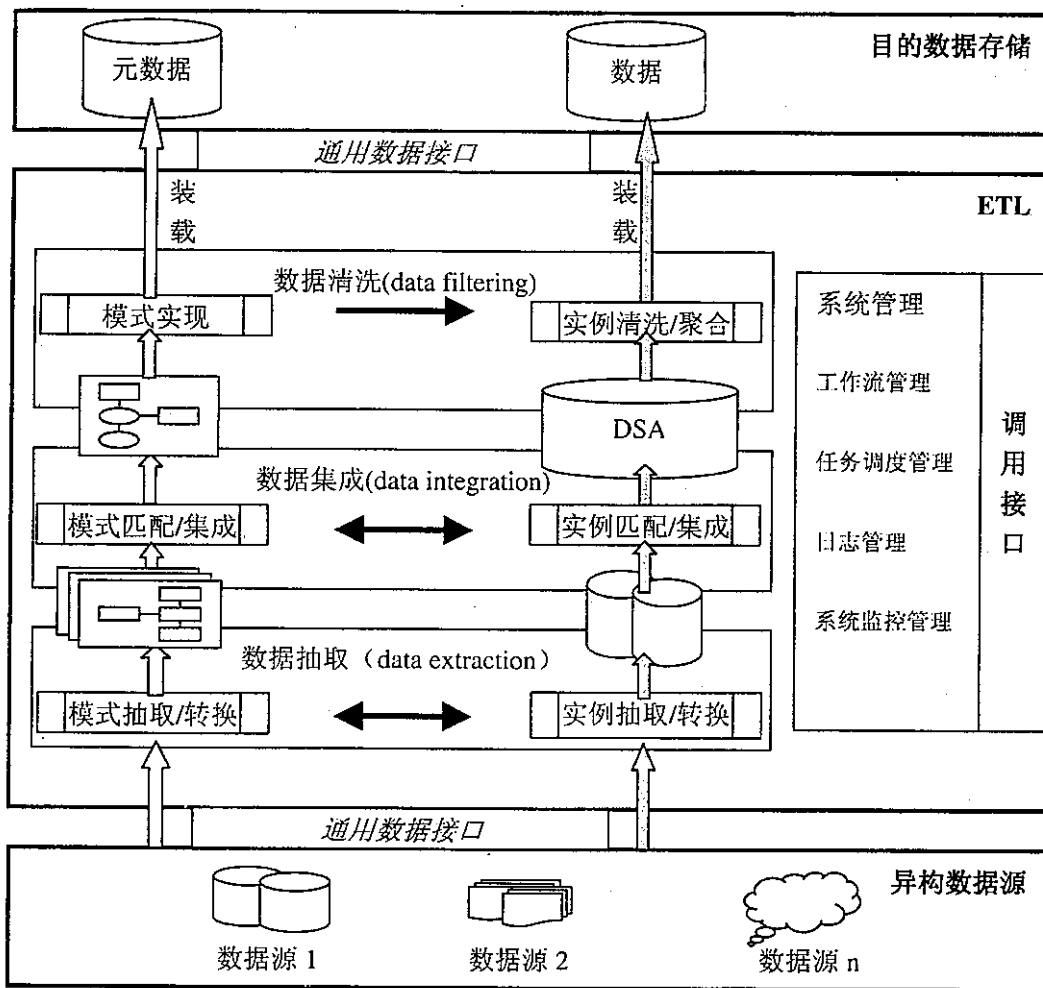
图 1 ETL 的体系结构图
